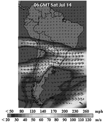
Esquema de las corrientes en chorro
