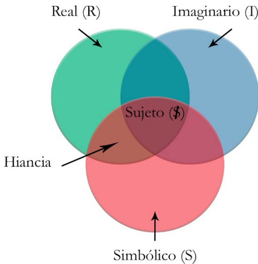
Nudo Borromeo
